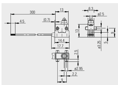
U Cable 300 long
